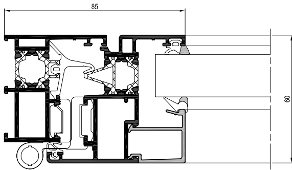
Sezione orizzontale
