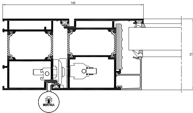
Sezione orizzontale
